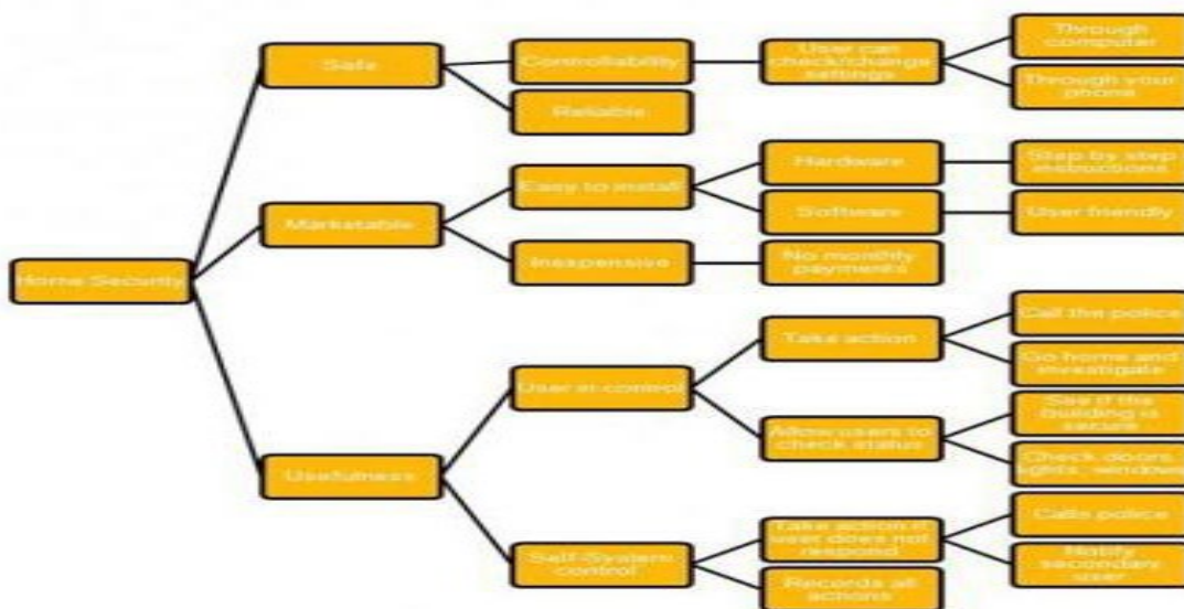
Рисунок 1. «Дерево» целей.
