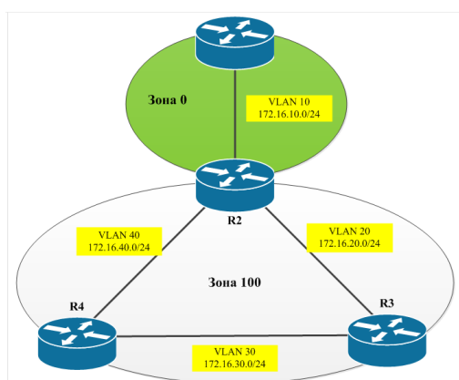
Рисунок 2 - Логическая топология
