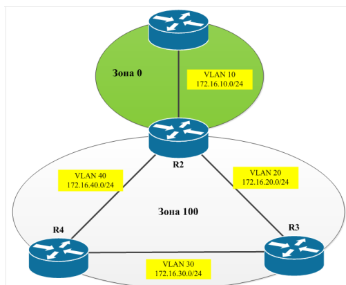
Рисунок 2 - Логическая топология
